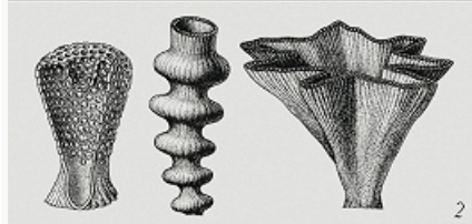
Археоциаты: 1 – сечение скелетов; 2 – внешний вид (реконструкция).
